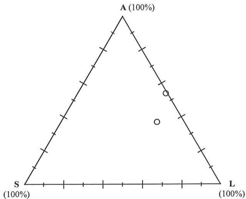
Figura 2.5 - Composizione granulometrica del terreno T2: Argilla con limo
