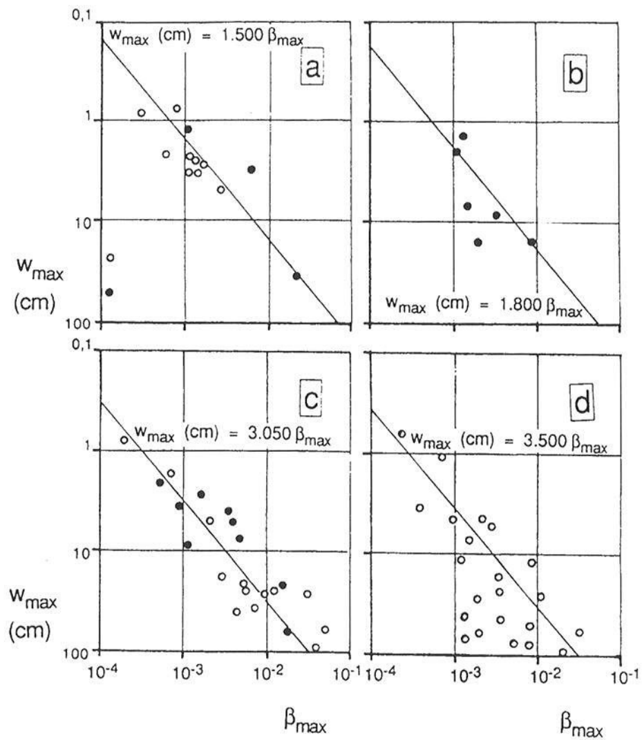
Figura 3.14 - Correlazione tra cedimenti assoluti massimi e distorsioni angolari massime.
