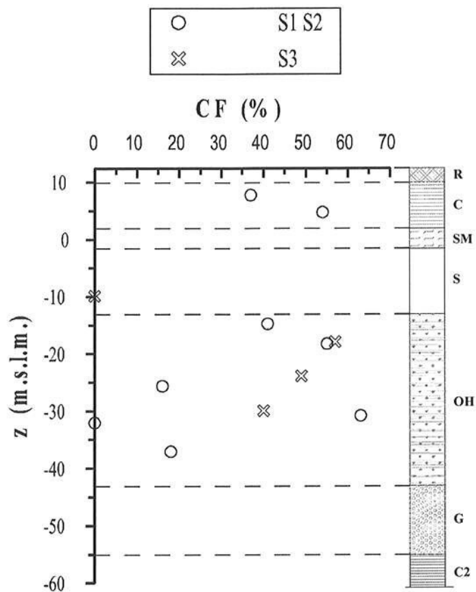
Figura 2.4 - Andamento della frazione argillosa con la profondità
