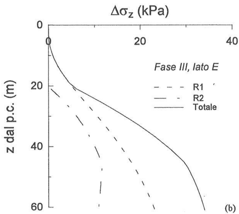
Figura 3.16 Incrementi di tensione verticale indotti nella fase III; (a) lato W e (b) lato E
